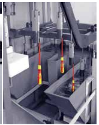
高電壓測試
