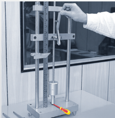
撞擊測試
