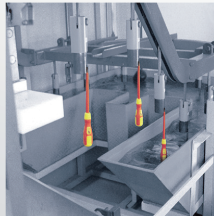
高電壓測試
